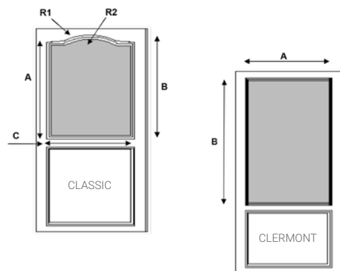
DIMENSION OCULUS MODÈLE CLERMONT
