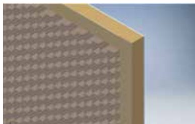
Âme alvéolaire
